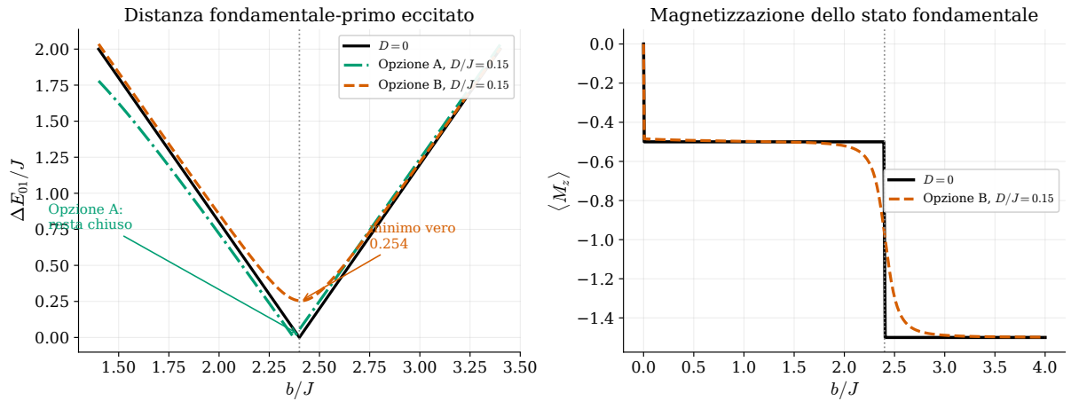
Figura 5: Sinistra: distanza fondamentale–primo eccitato, D = 0 contro le due opzioni di DM ( D/J = 0.15 ). L’Opzione A resta indistinguibile da D = 0 esattamente al punto critico; l’Opzione B apre un gap minimo vero, 0.254, spostato a b/J = 2.407 . Destra: magnetizzazione dello stato fondamentale, D = 0 contro Opzione B: il salto netto diventa un crossover continuo.
