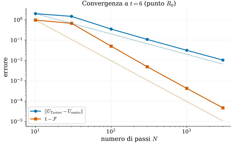
Figura 10: Errore a t = 6 (punto R_0 ), scala doppio-logaritmica. Le rette punteggiate sono le pendenze asymptotiche attese ( -1 per la norma dell'operatore, -2 per 1 - \mathcal{F} ).
