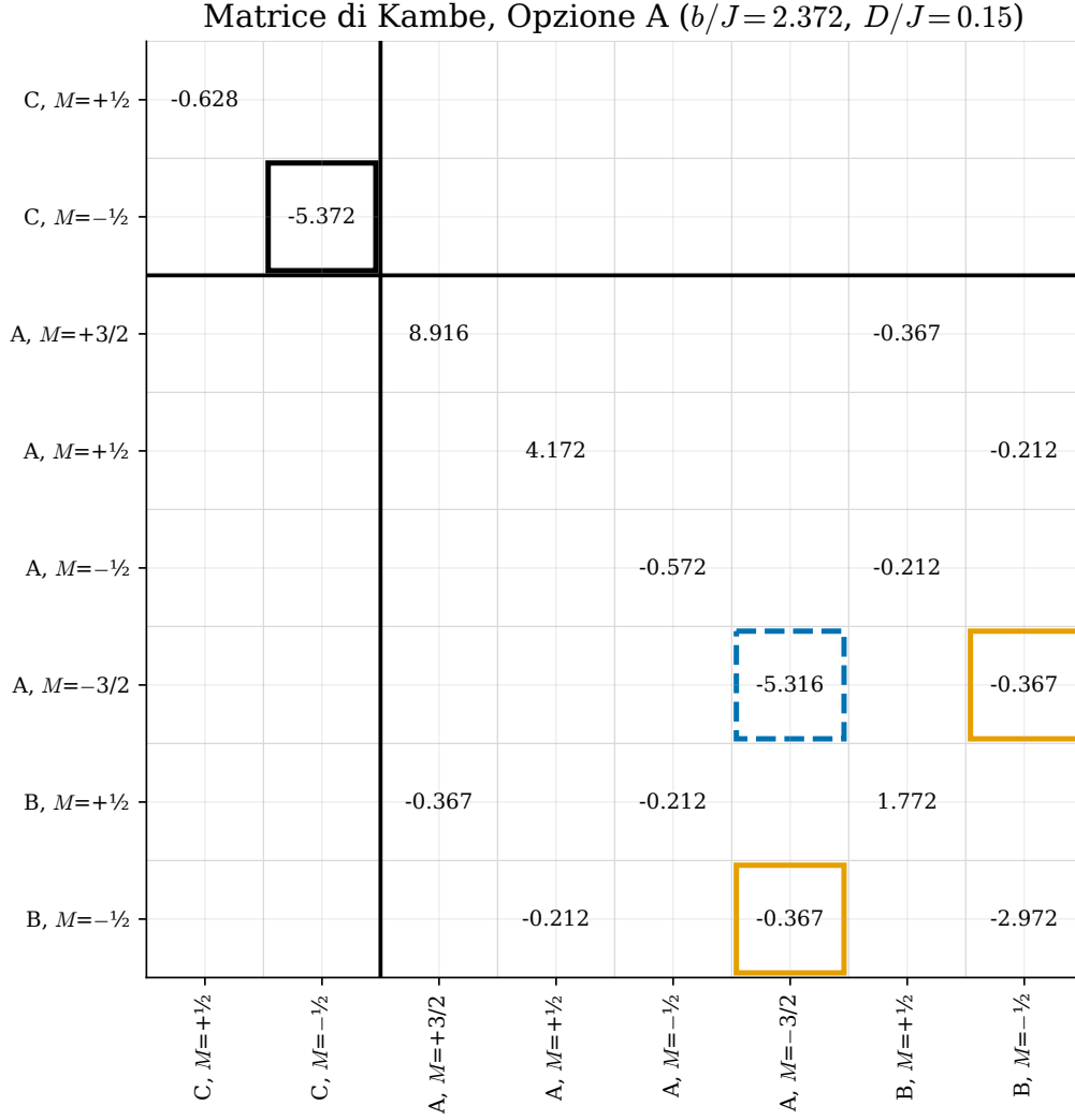
Figura 4: La stessa matrice di Figura 2 (Opzione A, b/J = 2.372 , D/J = 0.15 ), qui con i valori numerici. Riquadro nero: C(M=-1/2) — il ramo nero di Figura 3, comune a entrambi gli incroci. Riquadro blu tratteggiato: A(M=-3/2) puro — il ramo blu tratteggiato di Figura 3, il vecchio incrocio. Riquadri arancio: l'accoppiamento A(M=-3/2) \leftrightarrow B(M=-1/2) , -0.367 , l'unico elemento diverso da zero su quella riga/colonna: lo stato più basso del blocco 6 \times 6 a questo punto è per il 97.7% A(M=-3/2) e per il 2.3% B(M=-1/2) , miscelati esattamente da questo elemento — il ramo arancio di Figura 3, il nuovo incrocio.
